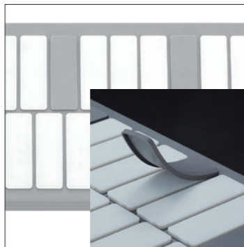
スケール設定に合わせて脱着し、黒鍵をブルーピング表示できる「ギャップキャップ」。
